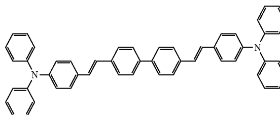
DPAVBi
