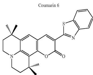
C545T
