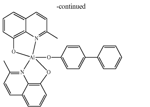
BAlq
