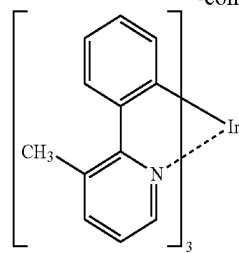
PhGD
